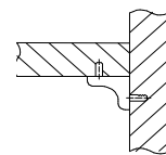
Полкодержатель фиксирующий
